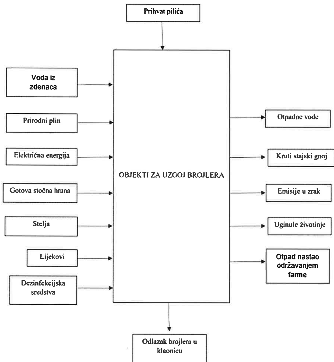
Prilog 2. Blok dijagram tehnološkog procesa novog postrojenja za intenzivan uzgoj peradi Farma Veliki Pažut
